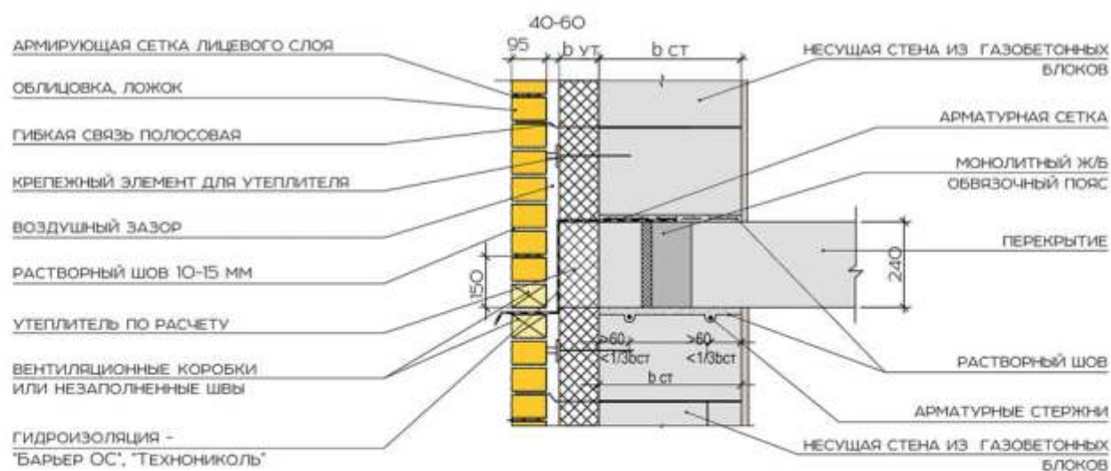
Узел 4.8 Опираение межэтажных перекрытий на газобетонную кладку с облицовкой и утеплителем
