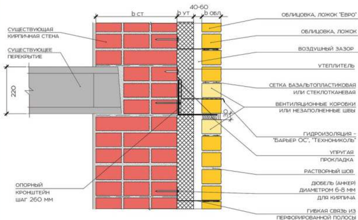
Узел 7.12 Устройство облицовки с расщечкой металлическими кронштейнами в уровне перекрытия
