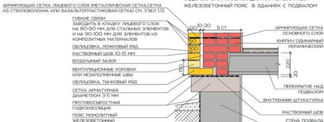
Узел 1.14 ОпираНИЕ кладки на монолитный ЖЕЛЕЗОБЕТОННЫЙ ПОЯС в зданиях с подвалом
