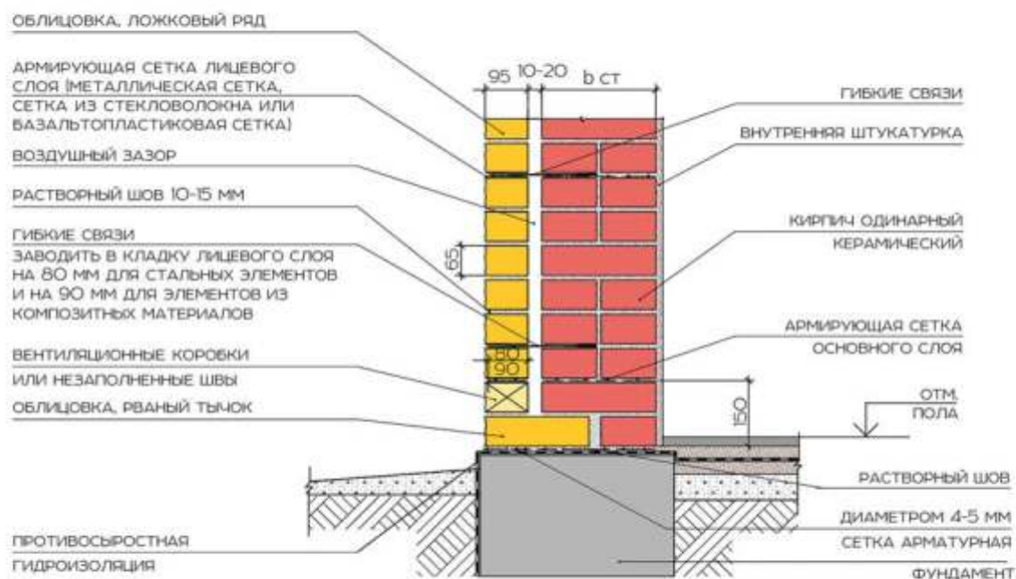
Узел 1.17 Опираение кладки на бетонный фундамент
