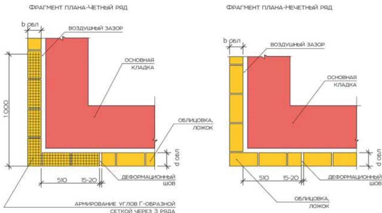
Узел 8.1 Порядовая перевязка лицевого слоя на углах
