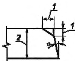
1 — размер фаски; 2 — толщина плиты; \alpha — угол наклона
