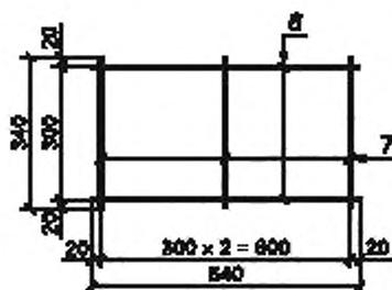
Рисунок Б.12 — Арматурная сетка С10
