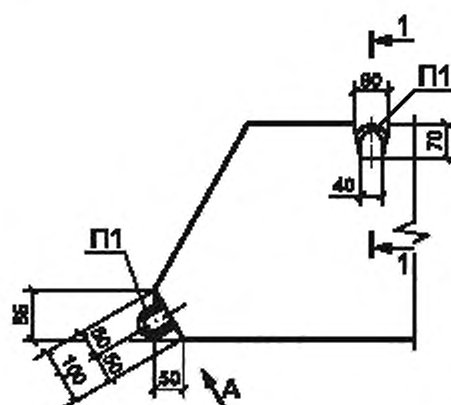
Рисунок Б.1 — Детали установки петель П1
