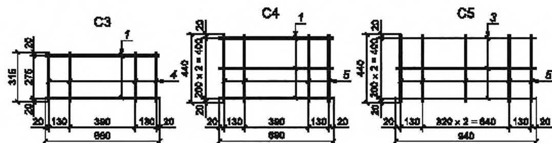
Рисунок Б.9 — Арматурные сетки C3, C4, C5
