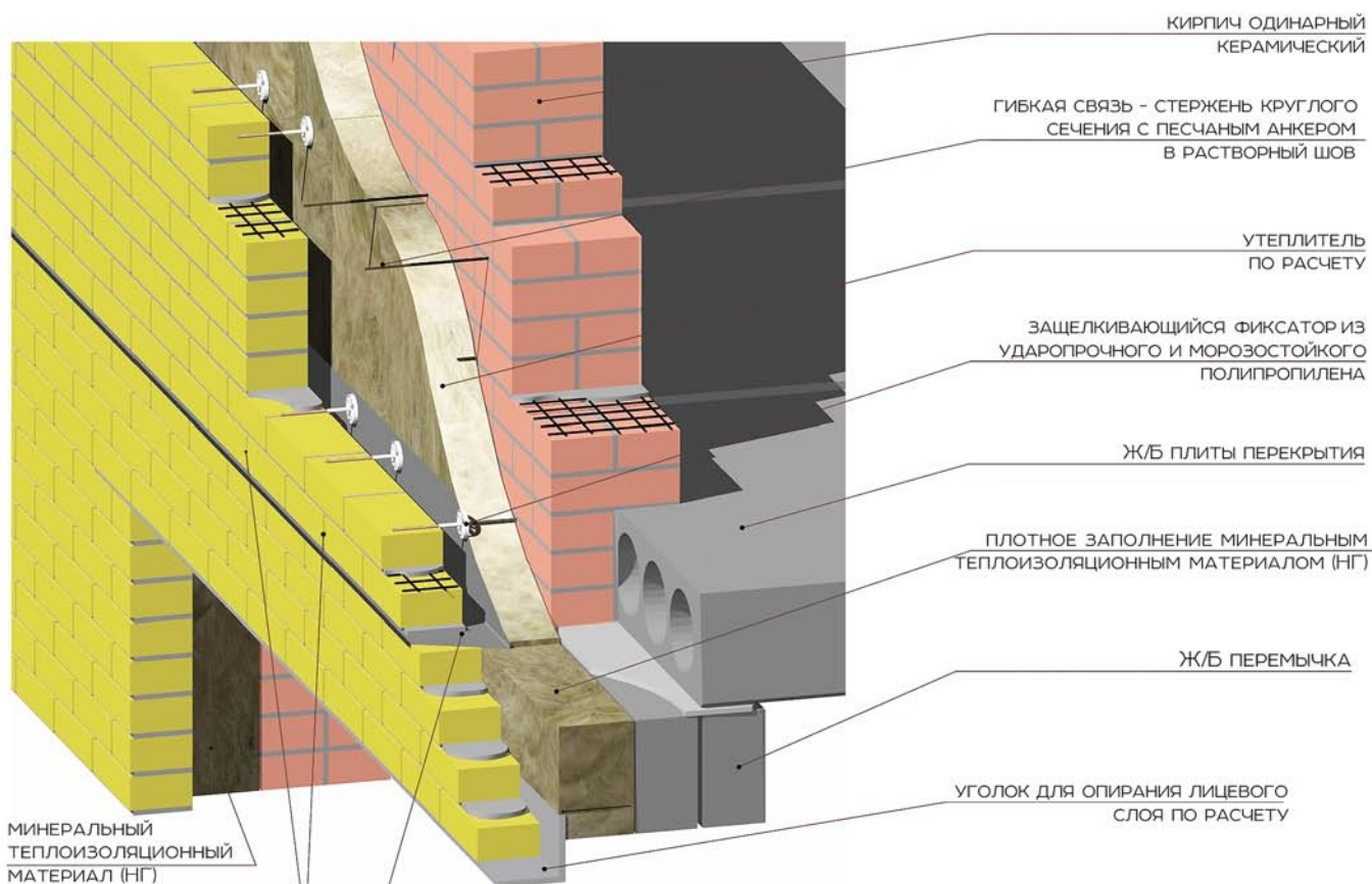
Узел 5.2 Облицовка простенка и устройство перемычки в облицовочном слое
